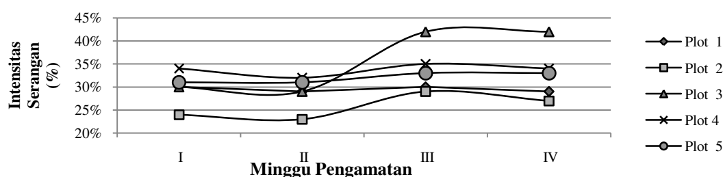
Gambar 1. Intensitas Serangan Helopeltis spp. pada Buah Kakao yang Diaplikasikan Cendawan Aspergillus sp. dengan Konsentrasi 10^5 spora/ml.
