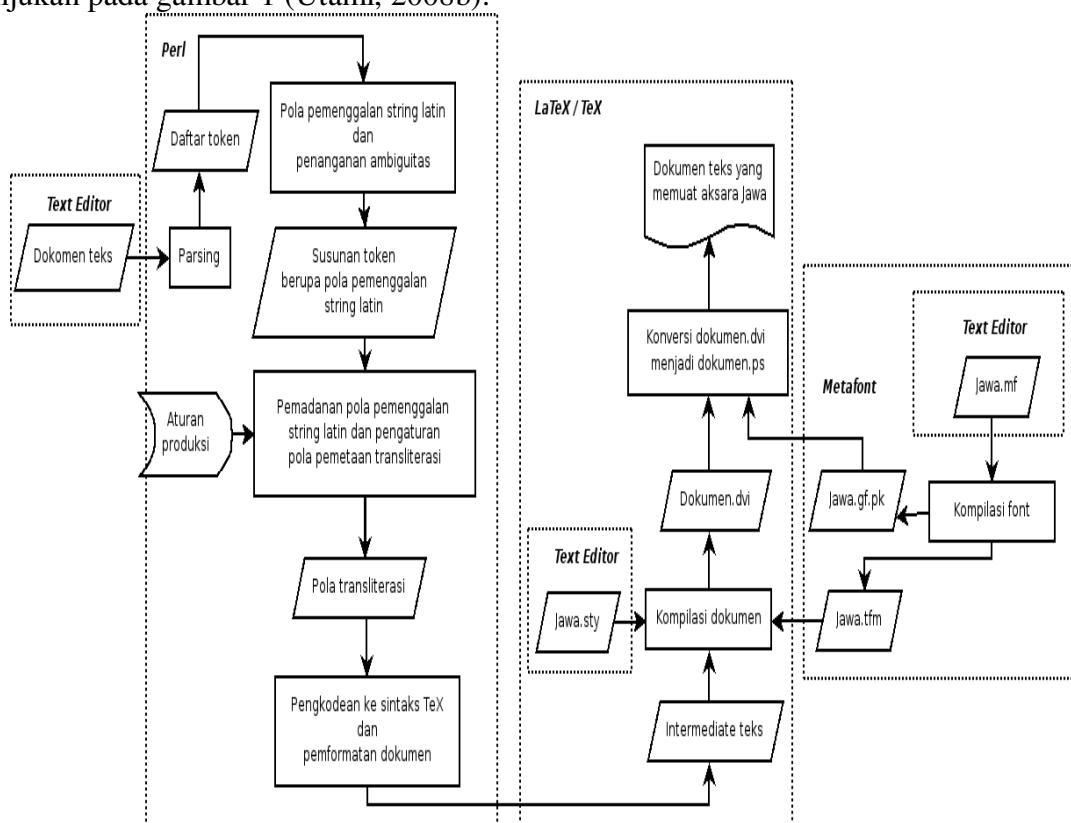
Gambar 1: Bagan proses transliterasi dokumen teks dalam karakter latin ke aksara Jawa
