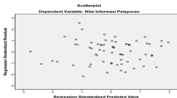
Gambar 2. Grafik heteroskedastisitas
