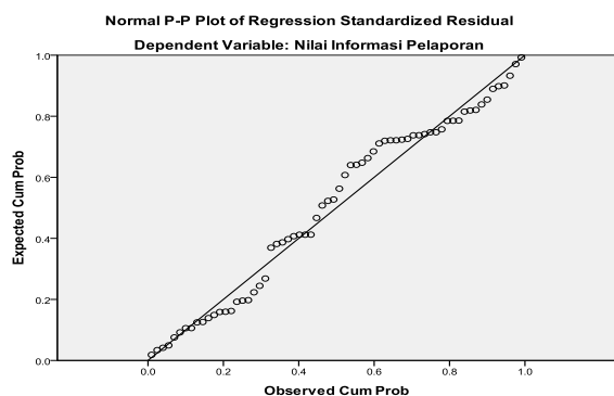
Gambar 1. Grafik Normalitas
