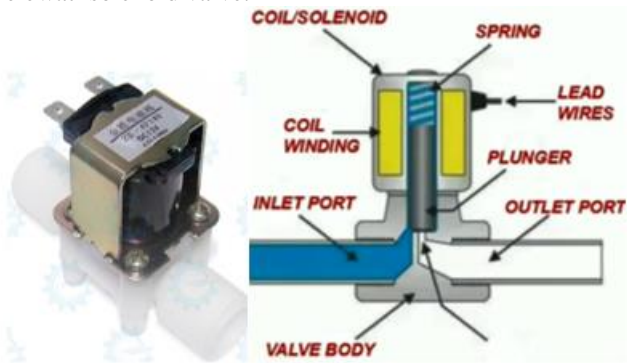
Gambar 2. Fisik dan bagian-bagian solenoid valve
