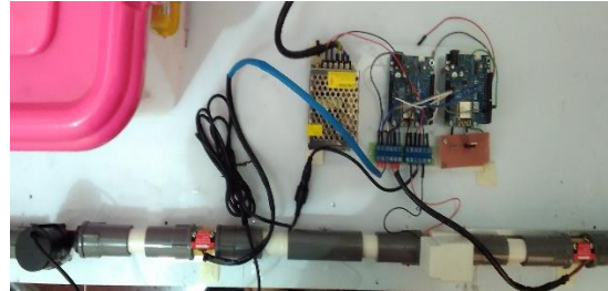
Gambar 10 Rangkaian alat untuk Monitoring Pemakaian Air
