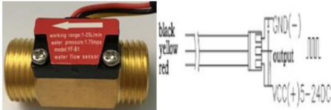
Gambar 1. Fisik dan skematik instalasi Water Flow Meter G1/2
