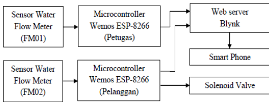
Gambar 8. Blok Diagram Alat
