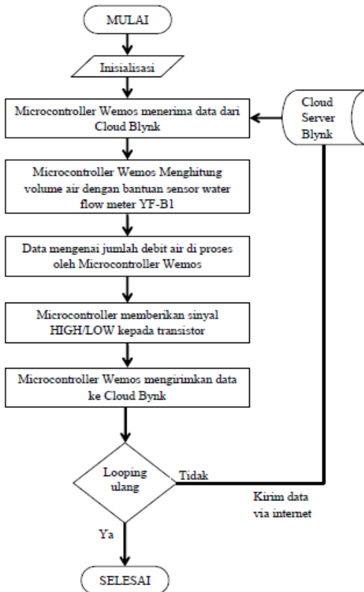
Gambar 9. Flowchart Sistem Perangkat Lunak
