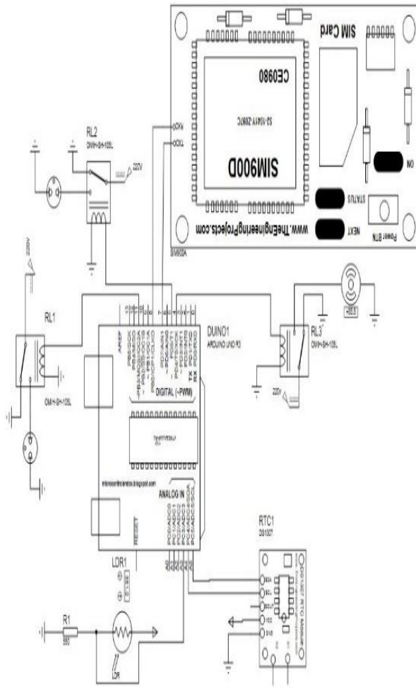
Gambar 5. Jalur kelistrikan
