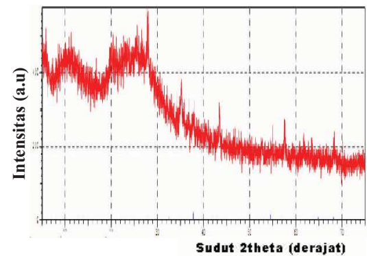
Gambar 3. Hasil XRD Zeolit Alam tanpa Kalsinasi.
