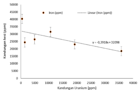
Gambar 1. Grafik kandungan uranium terhadap kandungan besi dalam bijih uranium BM-179 Eko-Remaja Kalan Kalimantan Barat.
