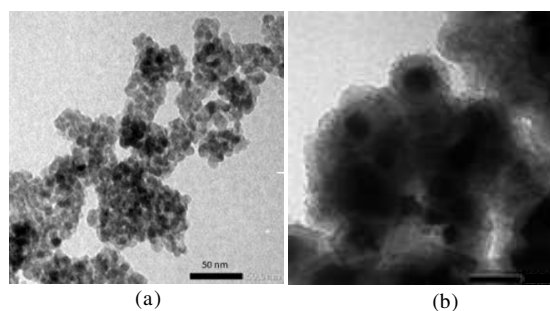
Gambar 5. Foto TEM (a) komposit Fe_3O_4-SiO_2-TiO_2 (b). perbesaran Gambar (a).
