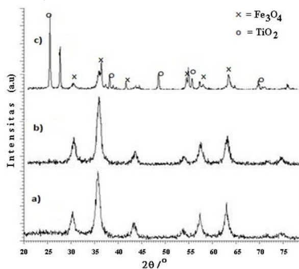
Gambar 1. Pola XRD (a). Fe_3O_4 , (b). Fe_3O_4-SiO_2 dan (c). Fe_3O_4-SiO_2-TiO_2
