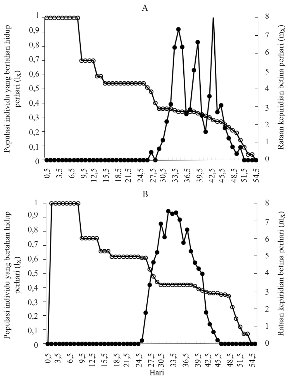
Gambar 1. Kurva lama hidup ( l_x : \circ ) dan rata-rata keperidian betina per hari ( m_x : \bullet ). A: Bemisia tabaci biotipe B; dan B: biotipe non-B pada tanaman cabai.
