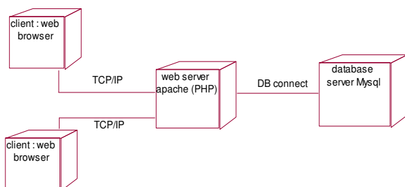
Gambar 26. Deployment diagram Aplikasi ujian PSB online
