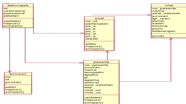
Gambar 24. Class diagram Aplikasi ujian online
