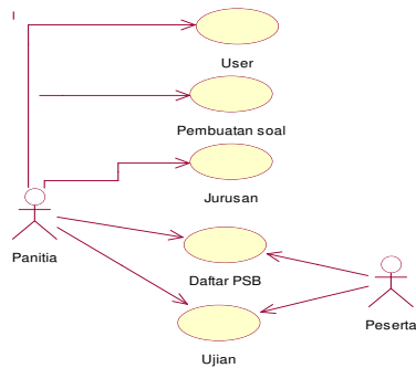
Gambar 8. Use case diagram yang diusulkan
