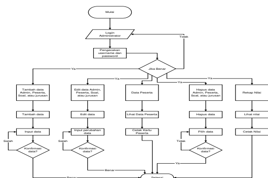
Gambar 2. Flowchart untuk admin
