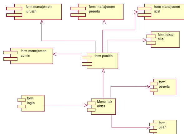
Gambar 25. Component diagram Aplikasi ujian PSB online
