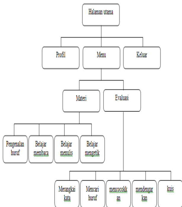
Gambar 4.2 Struktur Menu Utama
