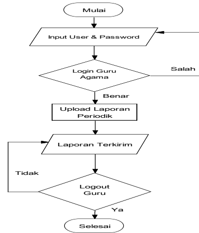
Gambar 3. Flowchart Pengiriman laporan Periodik untuk halaman Guru
