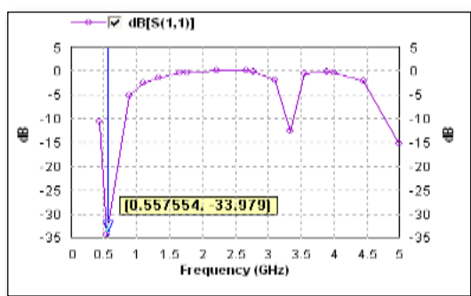
Fig.3: S11 Parameter
