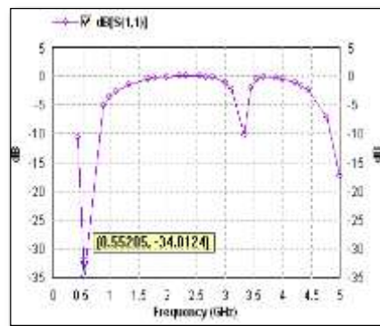
Fig.7: S11 parameter
