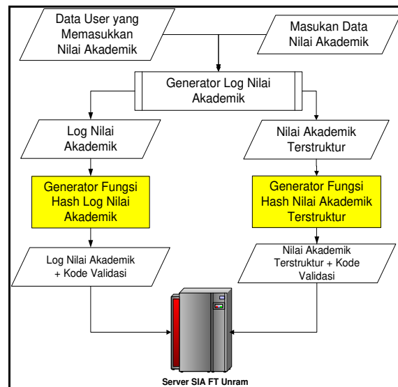
Gambar 2. Desain Sistem Pengamanan Data Nilai Akademik
