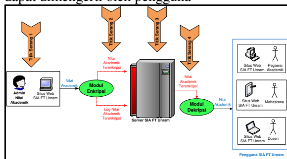
Gambar 1. Diagram Global Sistem Pengamanan Data Nilai Akademik pada SIA FT Unram
