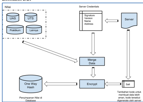
Gambar 3. Desain Sistem Enkripsi untuk Mengamankan Data Nilai Akademik
