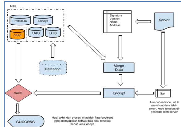
Gambar 4. Desain Sistem Validasi Data Nilai Akademik
