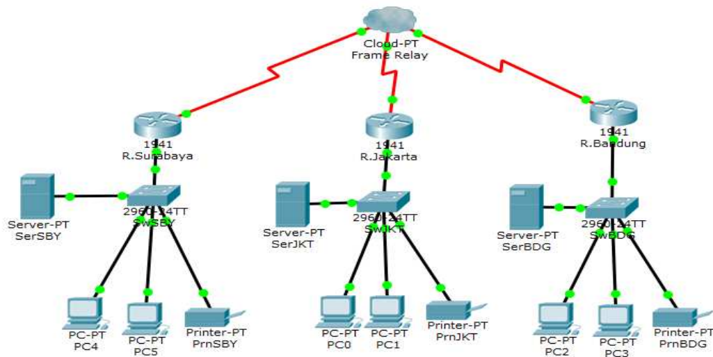
Gambar 2. Topologi WAN dengan frame relay PT. Eka Daya Unggul
