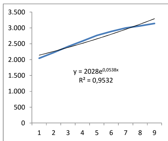
Gambar 4: Kurva model eksponensial penjualan energi listrik Penerangan Umum
