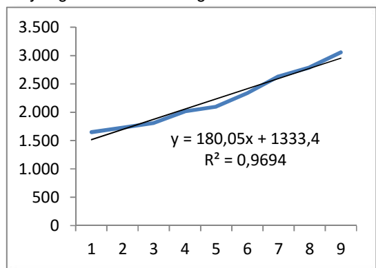
Gambar 6: Kurva model linier penjualan energi listrik Pemerintah
