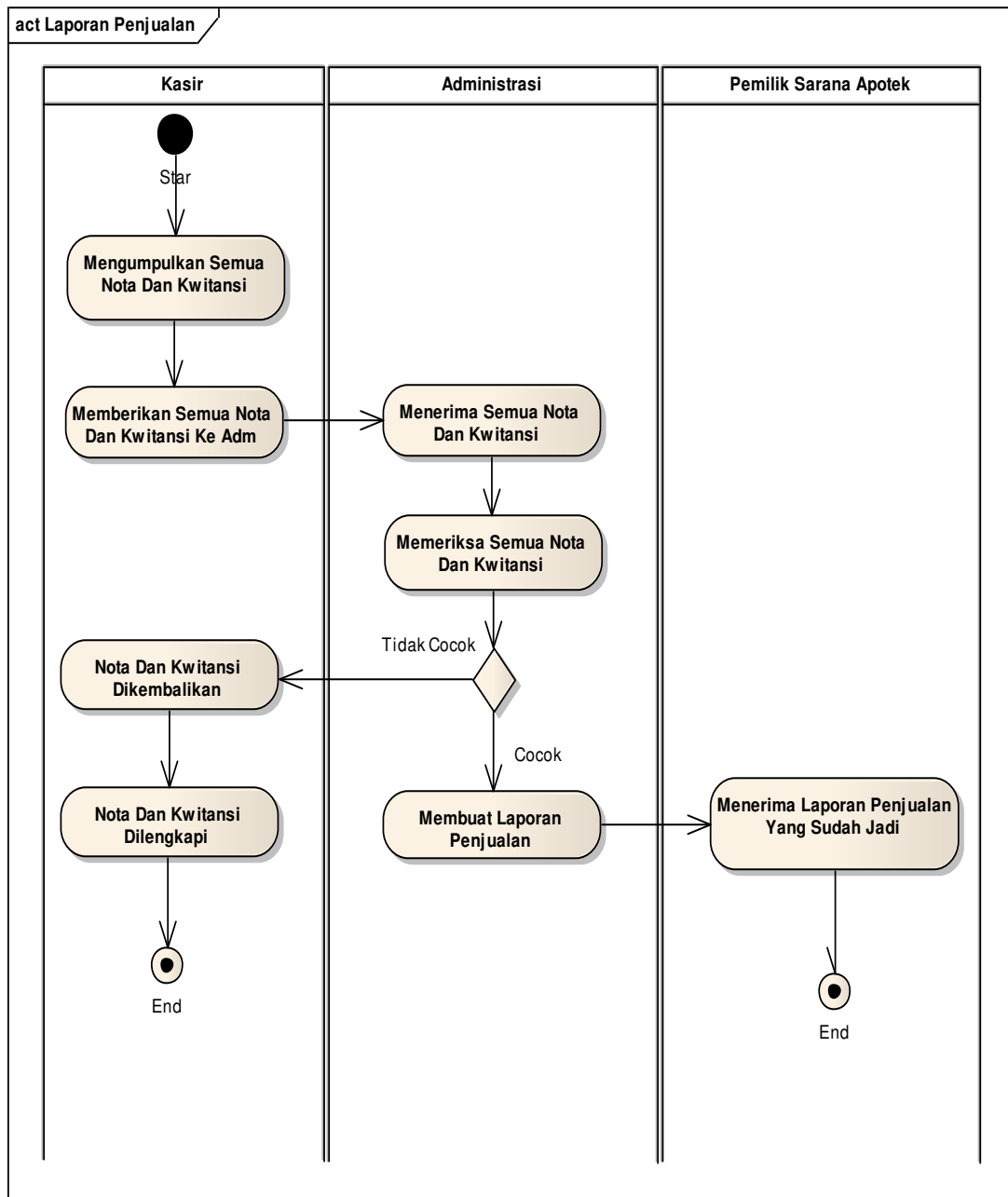
Gambar 3. Activity Diagram Pembuatan Laporan Penjualan Bulanan
