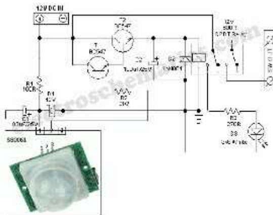
Gambar 2. Rangkaian Sensor Gerak
