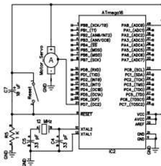
Gambar 3. Rangkaian Sistem Minimum Mikrokontroler Atmega16
