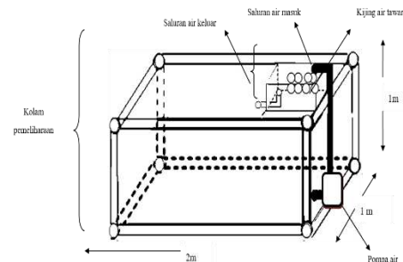
Gambar 1. Sketsa sistem resirkulasi dengan penambahan biofilter kijing air tawar
