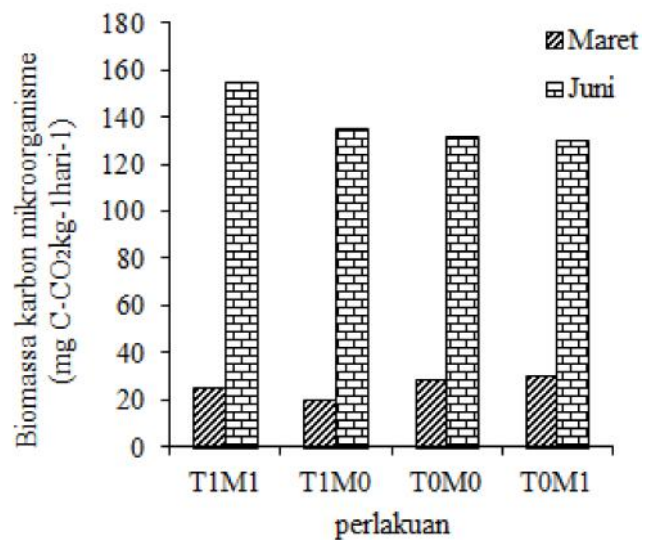
Gambar 2. Biomassa karbon mikroorganisme tanah (mg C-CO 2 kg -1 hari -1 ) di Pertanian tebu PT GMP pada pengamatan 9 BST dan 12 BST 2014. (T 0 = tanpa olah tanah, T 1 = olah tanah intensif, M 0 = tanpa mulsa bagas, M 1 = mulsa bagas 80 t ha -1 , tongkat diatas menunjukkan standar deviasi)
