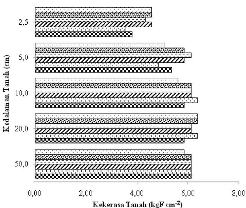
Gambar 1. Kekerasan tanah pada berbagai sistem pengolahan tanah dan pemberian residu pemupukan nitrogen, N_0 = tanpa residu pupuk, N_1 = residu pupuk 100 \text{ kg N ha}^{-1} , TOT = tanpa olah tanah, OTM = olah tanah minimum, OTI = olah tanah intensif □ = TOTN 0 , ▨ = TOTN 1 , ▩ = OTMN 0 , ▧ = OTMN 1 , ▦ = OTIN 0 , ▤ = OTIN 1
