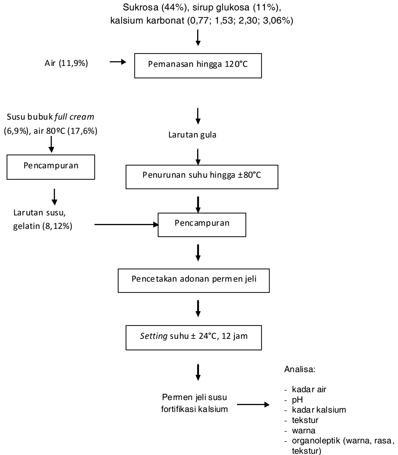
Gambar 1. Diagram Alir Pembuatan Permen Jeli Susu Fortifikasi Kalsium
