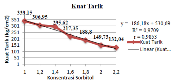
Gambar 2. Pengaruh Penambahan Sorbitol terhadap Kuat Tarik Edible Film
