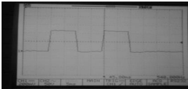
Gambar 20. Sinyal Yang Dipancarkan Remote Unit
