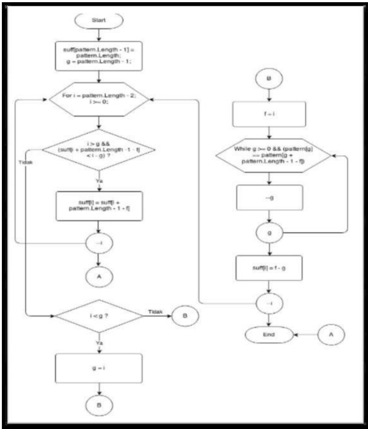
Gambar 7 Alur kerja perulangan suffix
