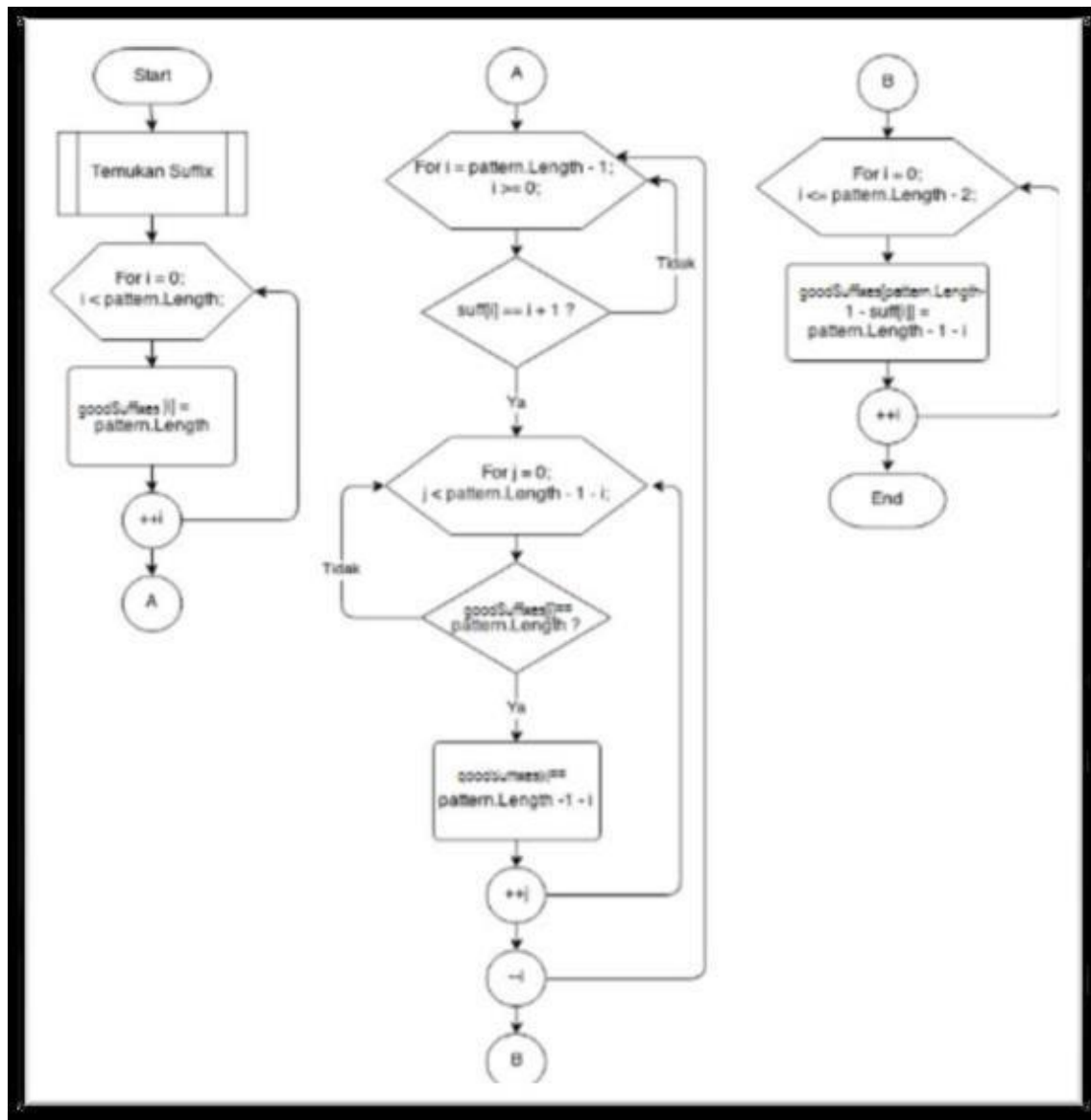
Gambar 6 Flowchart alur kerja
