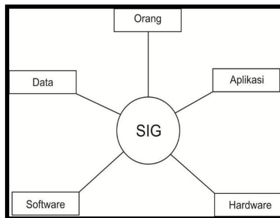
Gambar 2 Komponen-Komponen SIG
