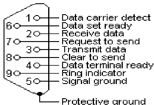
Gambar 2. Penggunaan Pin pada RS232 Pin 9
