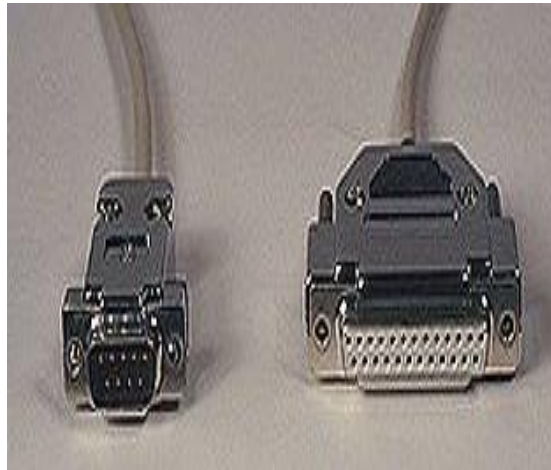
Gambar 1. RS232 – Pin 9 (kiri) dan Pin 25 (kanan)
