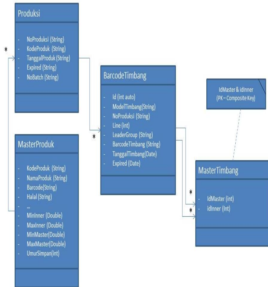
Gambar 9. Class Diagram – Sistem aplikasi Barcode Timbangan
