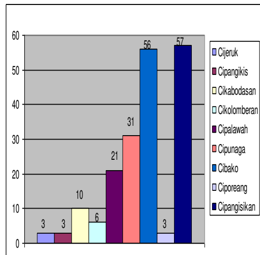
Gambar 2. Penyebaran Rafflesia patma di CA Leuweung Sancang
