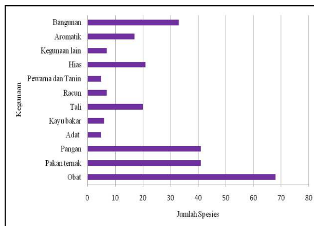
Gambar 4. Kelompok kegunaan pada masyarakat Buaq
