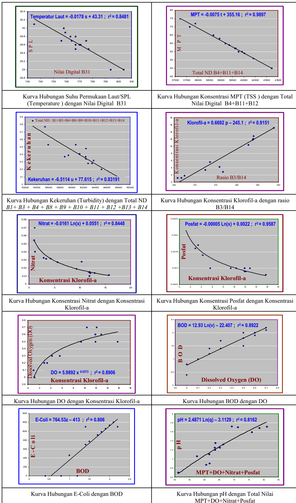
Gambar 3. Kurva Hubungan beberapa parameter Kualitas Air
