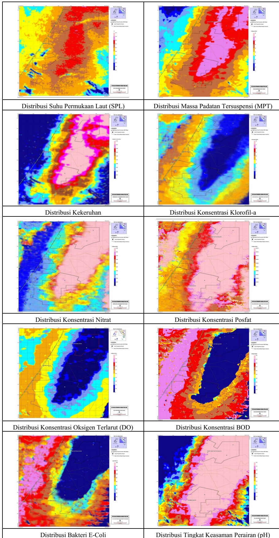
Gambar 4. Distribusi Beberapa Parameter Kualitas Air Berdasarkan Data Citra Satelit MODIS
