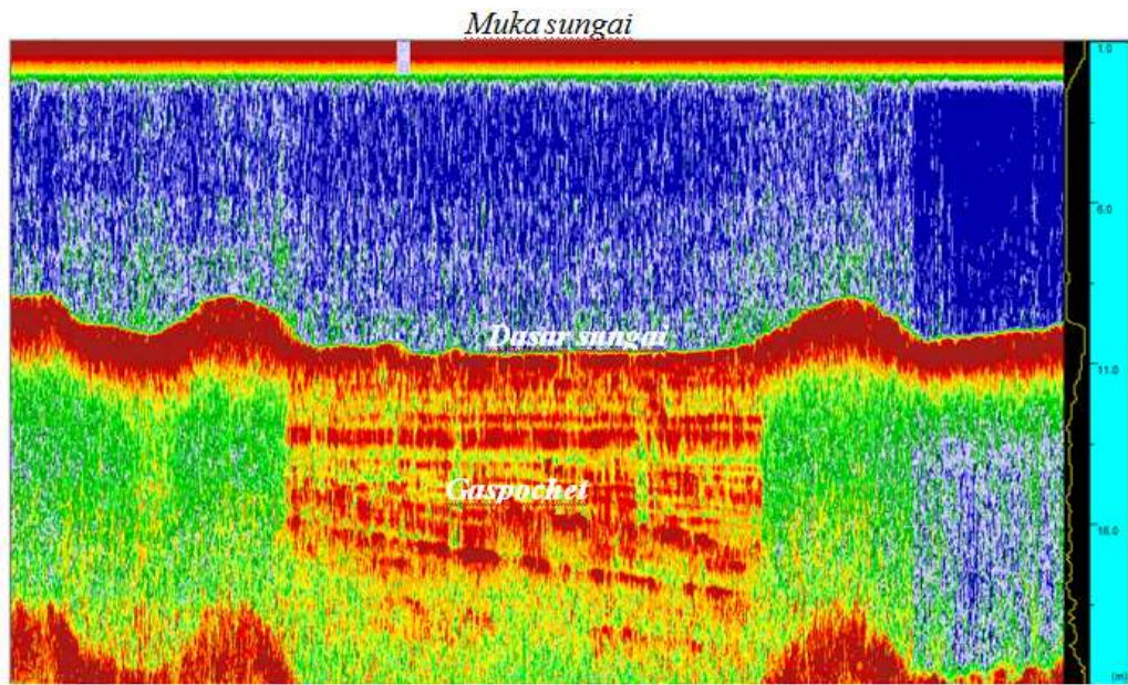
Gambar 7. Rekaman Strata Box dengan kantong gas (gas pocket) di Lintasan CR-02.
