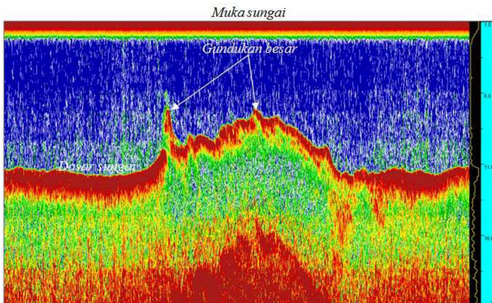
Gambar 10. Rekaman Strata Box yang memperlihatkan adanya Gundukan besar-kecil di Lintasan CR-01.
