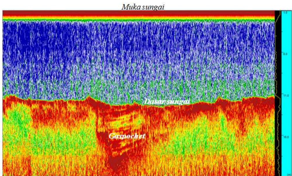
Gambar 8. Rekaman Strata Box dengan kantong gas (gas pocket) di Lintasan CR-01.
