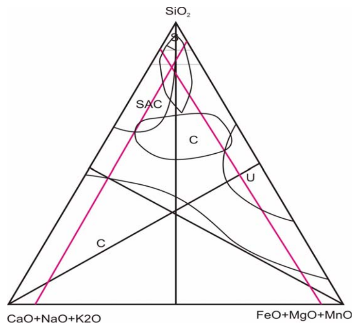
Gambar 3. Contoh salah satu hasil plotting dalam segitiga perbandingan antara data unsur SiO 2 , CaO + Na 2 O + K 2 O, dan FeO + MgO + MnO
