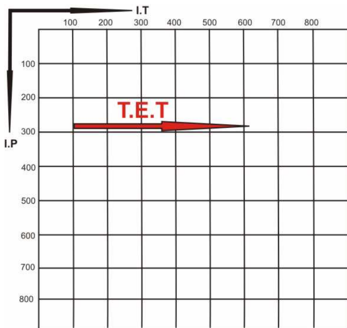
Gambar 5. Trend Umum Evolusi Mineral Zirkon Di Daerah Penelitian (I.T = Indikasi terhadap temperatur, I.P = Indikasi terhadap tekanan )
