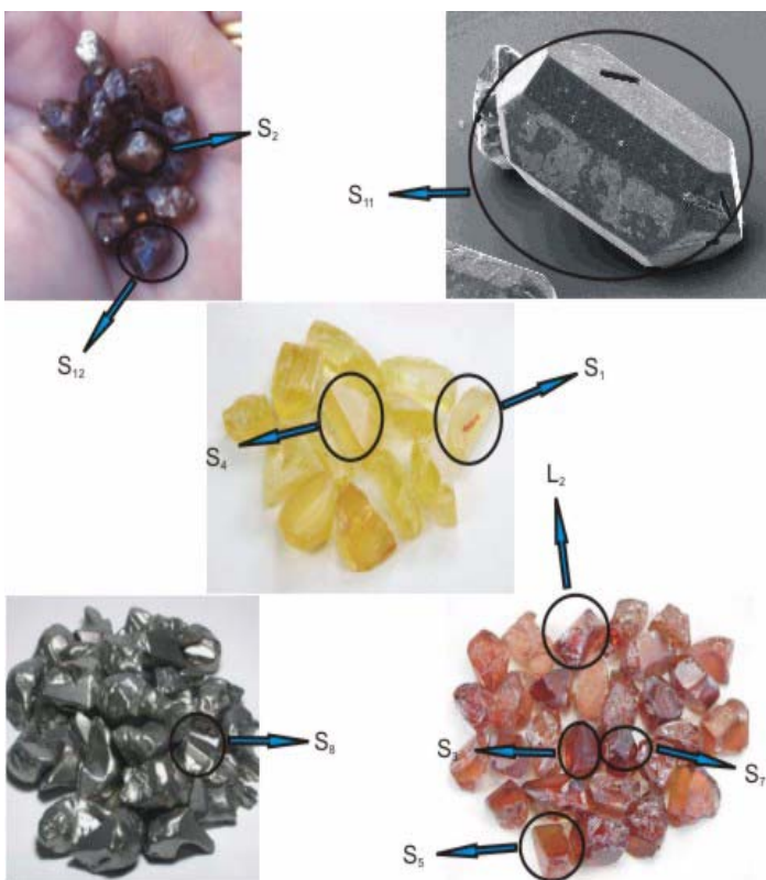
Gambar 4. Contoh bentuk-bentuk Piramid Zirkon Hasil Pemisahan menurut Pupin, (1980)
