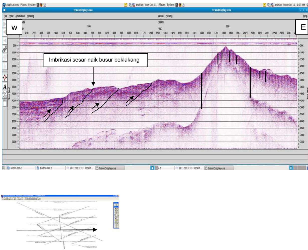
Gambar 4. Imbrikasi sesar naik busur belakng (back arc thrust) di daerah penelitian
