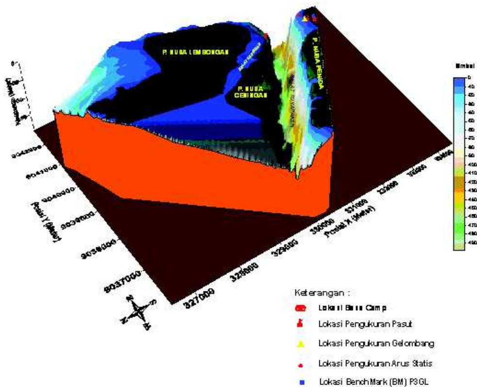
Gambar 5. Gambaran 3 dimensi morfologi dasar laut di Selat Toyopakeh - Nusa Penida, Bali
