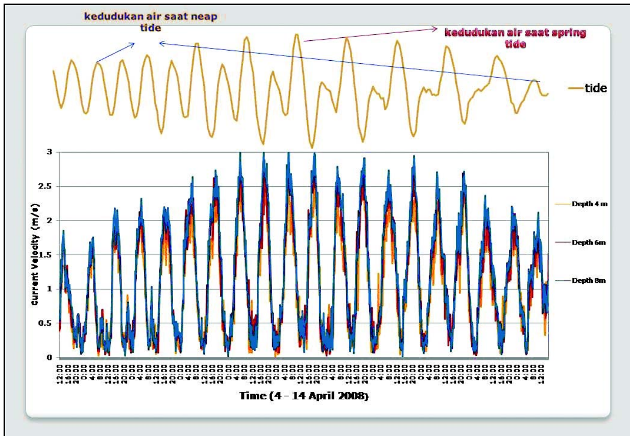
Gambar 2. Kecepatan arus pada kedalaman 4, 6 dan 8 meter dalam kondisi pasang purnama (spring tide) dan surut perbani (neap tide), hasil pengukuran arus di Selat Toyapakeh, Nusa Penida (Yuningsih, dkk, 2008).
