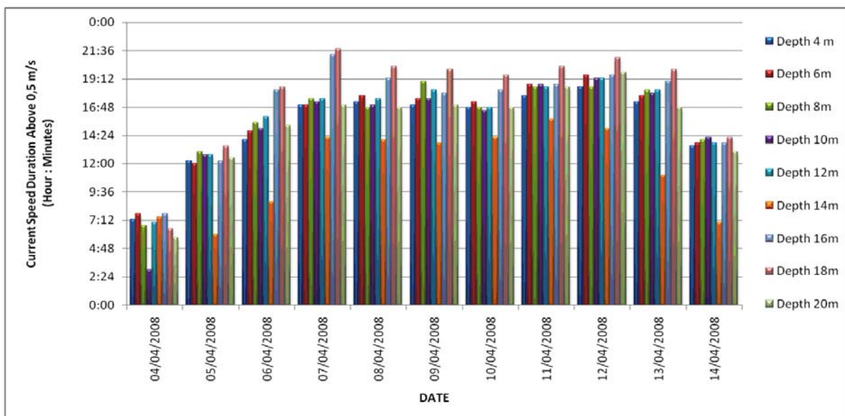
Gambar 3. Grafik durasi kecepatan arus di atas 0.5 m/det (Yuningsih, dkk.,2008)
