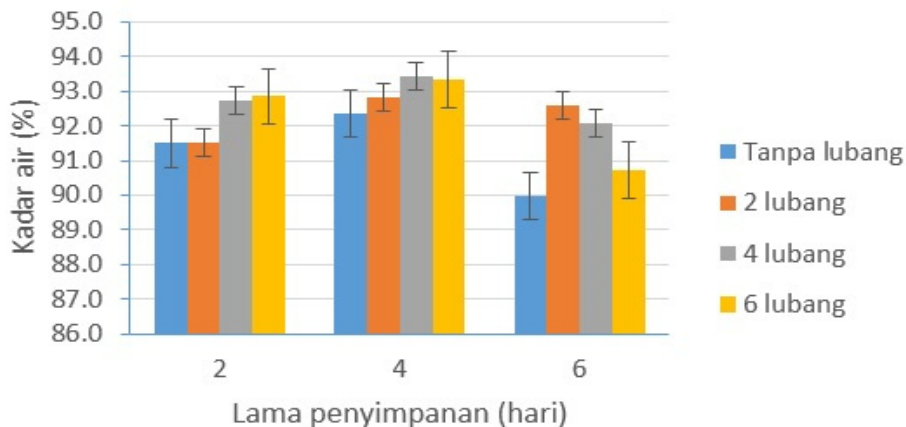
Gambar 1b. Pengaruh jumlah lubang perforasi kemasan terhadap kadar air sawi hijau selama penyimpanan pada suhu 5°C
