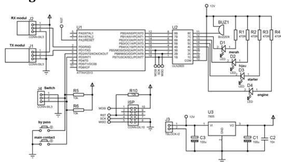
Gambar 9. Rangkaian keseluruhan pada pengaman motor
