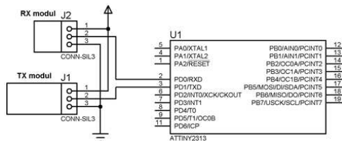
Gambar 7. Rangkaian modul TX dan RX pada rangkaian pengaman motor
