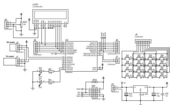
Gambar 10. Rangkaian keseluruhan pada remote
