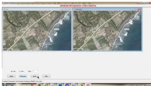
Gambar 7. Hasil eksekusi
