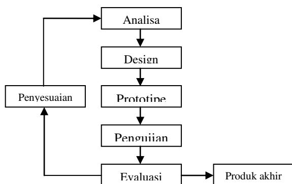
Gambar 3. Tahapan penelitian
