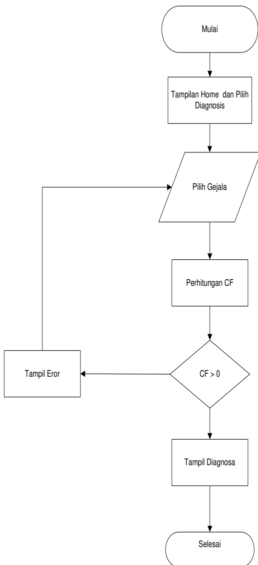
Gambar 4. Rancangan Algoritma
