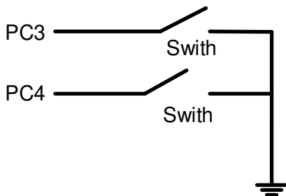
Sumber : Rosano, Yunita & Raharjo (2016) Gambar 6. Rangkaian Switch
