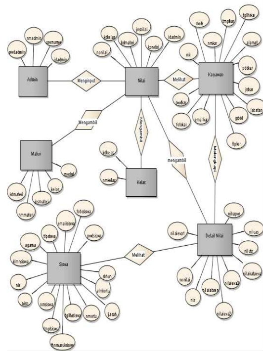
Sumber: Hasil Penelitian (2017) Gambar 6. ER Diagram Sisfo Akademik
