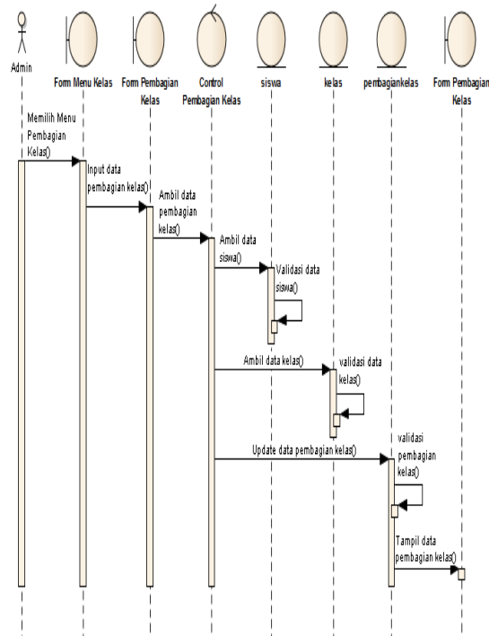
Sumber: Hasil Penelitian 2017 Gambar 4. Sequence Diagram Input Data Pembagian Kelas
