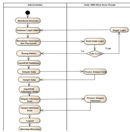
Sumber: Hasil Penelitian (2017) Gambar 3. Activity Diagram Sistem Siswa dan Sisfo
