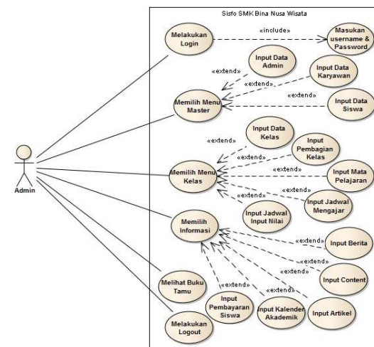
Sumber: Hasil Penelitian (2017) Gambar 2. Use Case Diagram Sistem Halaman Utama Siswa
