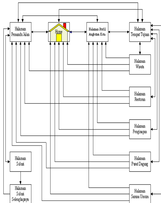
Gambar 4. Struktur Navigasi
