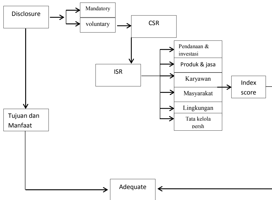
Gambar 1.1 kerangka pemikiran
