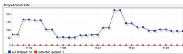
Gambar 6 Hasil deteksi serangan UDP flood
