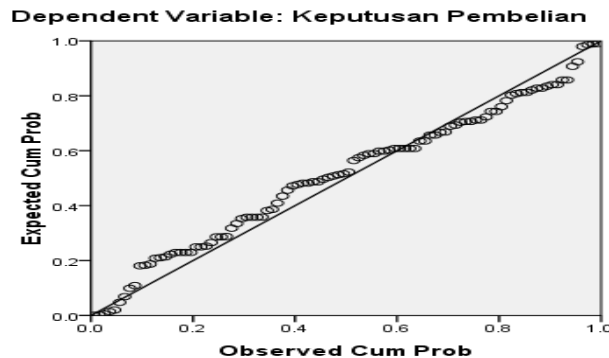
Gambar 3. Uji Normalitas
