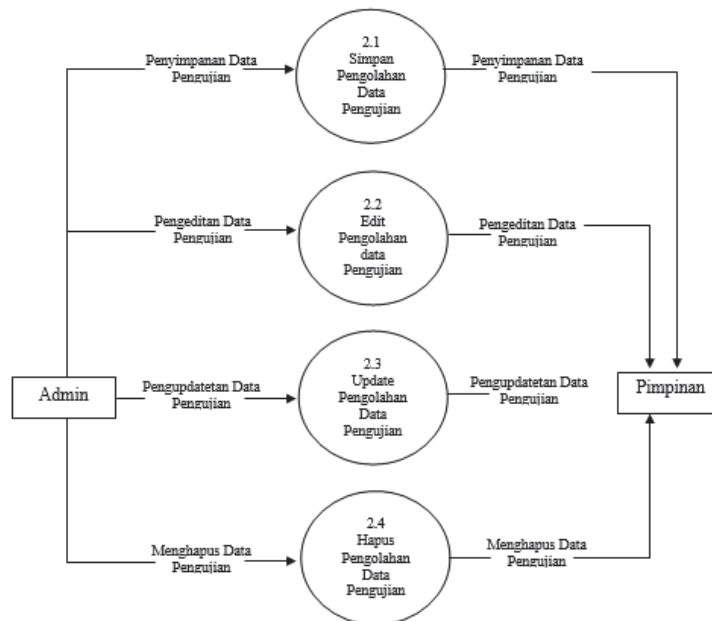
Gambar 6. DFD Level 2 untuk Proses 3 (Pengelolaan Data Pengujian)
