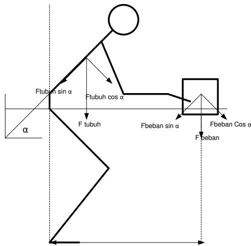
Gambar 2 Diagram benda bebas model punggung bawah (Iridiastadi & Yassierli, 2014)
