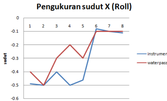
Gambar 7. Grafik Output sudut X (Roll)
