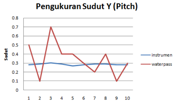
Gambar 8. Grafik Output sudut Y (Pitch)
