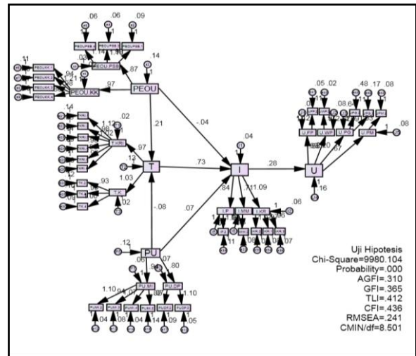
Gambar 3. Model SEM Tahap Awal
