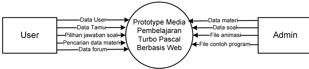
Gambar 2. Diagram Konteks Prototype Media Pembelajaran Pascal
