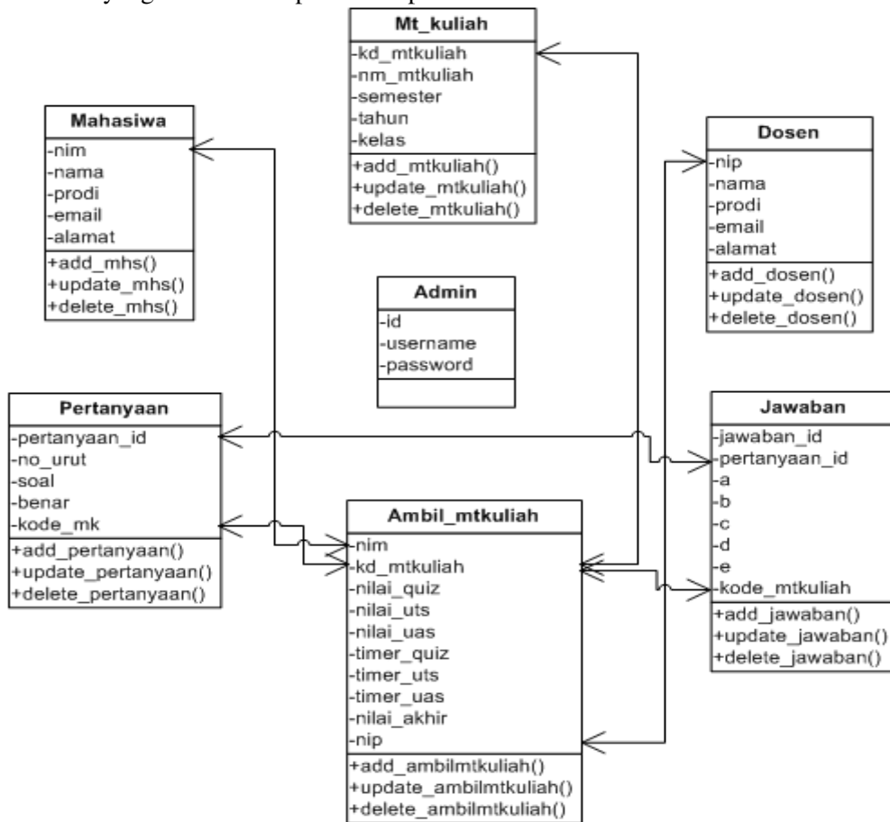
Gambar. 8. Kelas Diagram
