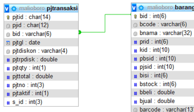
Gambar 1. Desain Database
